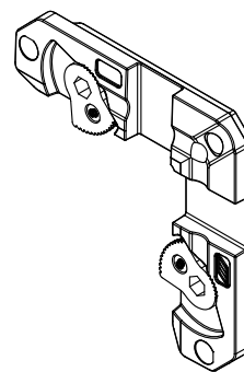
MONTAGGIO SQUADRETTA Profilo esterno Art. ARX.15.SQ Taglio a 45° o a 90° parti fisse
