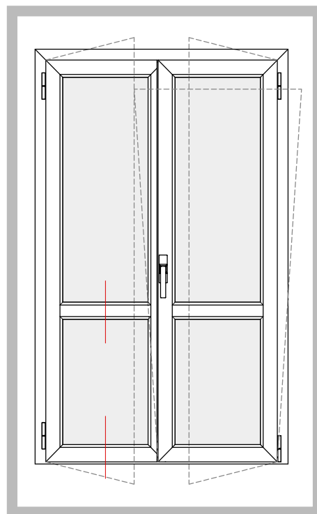
PORTA BALCONE A A DUE ANTE Anta MX603.202
