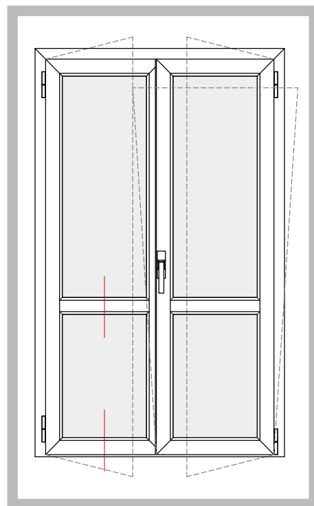
PORTA BALCONE A A DUE ANTE Anta MX603.201
